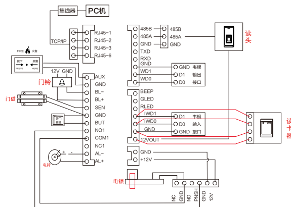
专用电源接线图
