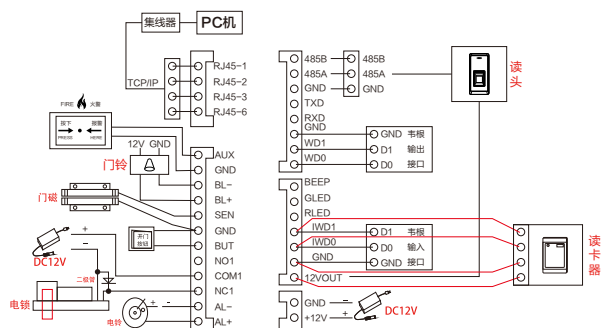
普通电源接线图
